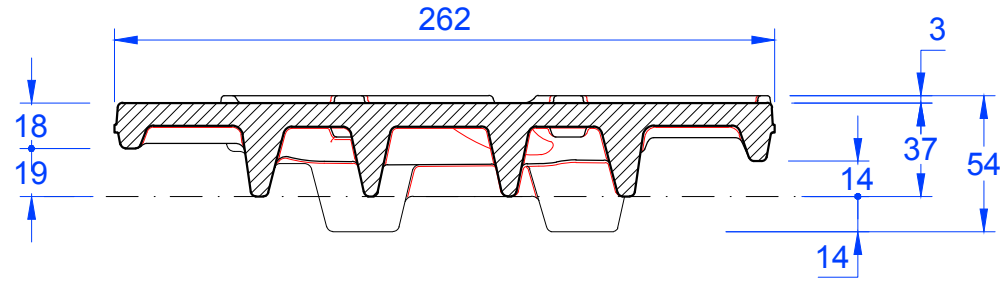
Schnitt A-A
