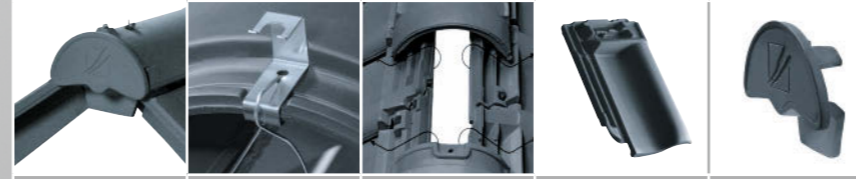
Firstabschluss „FIRSTFIX“ Luftzirkulation Firstanschluss-Lüfterziegel Firstendscheibe
